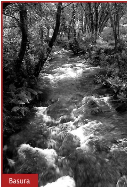
Patxiloketa
